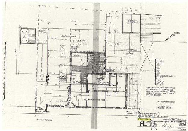
Grundriss Erdgeschoss
