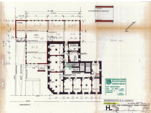
Grundriss Untergeschoss-Keller
