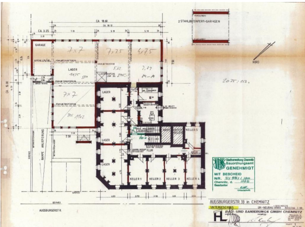
Grundriss Untergeschoss-Lager
